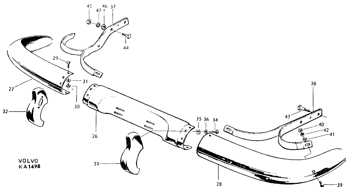
Bild nr 41 Stötfångare
