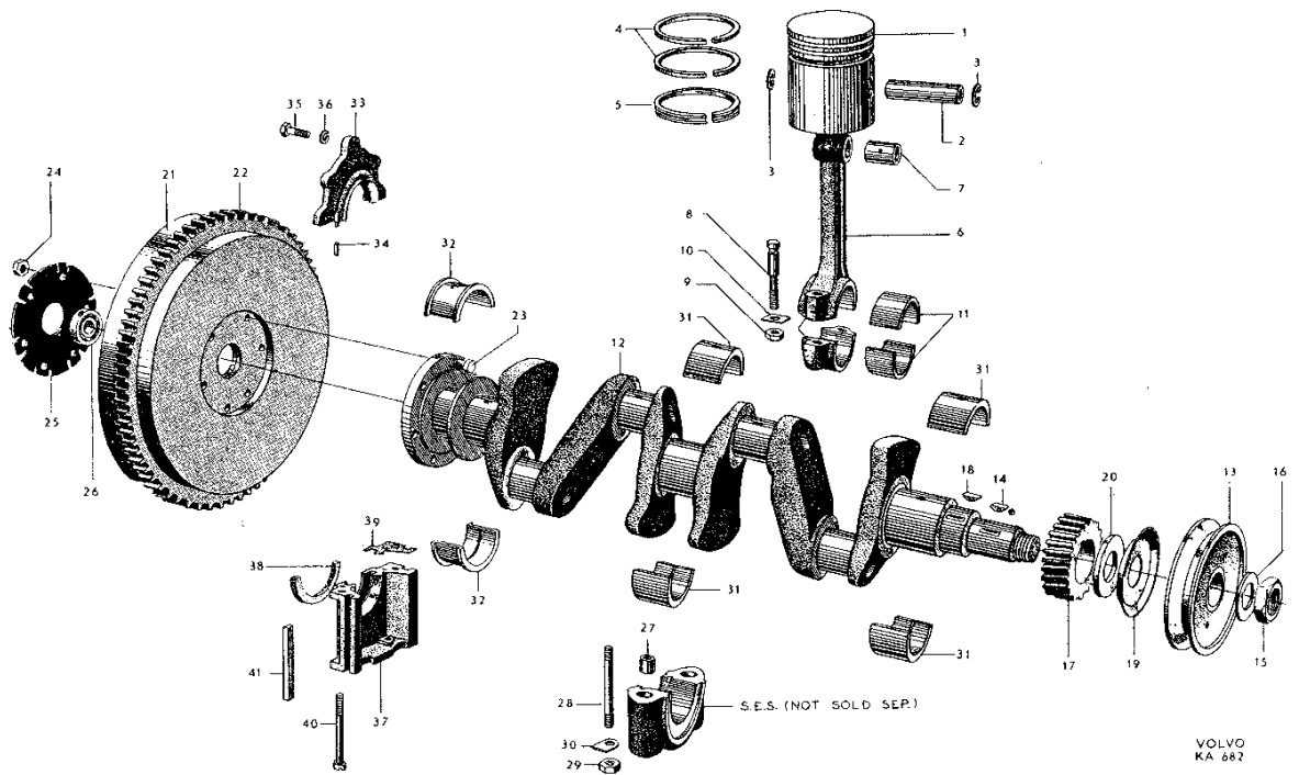
Bild nr 4 Vevrörelse
