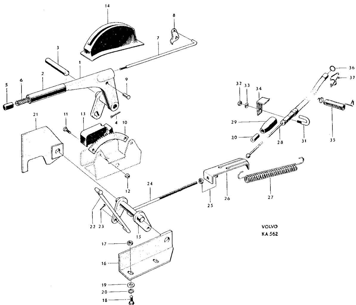
Bild nr 36 Handbroms
