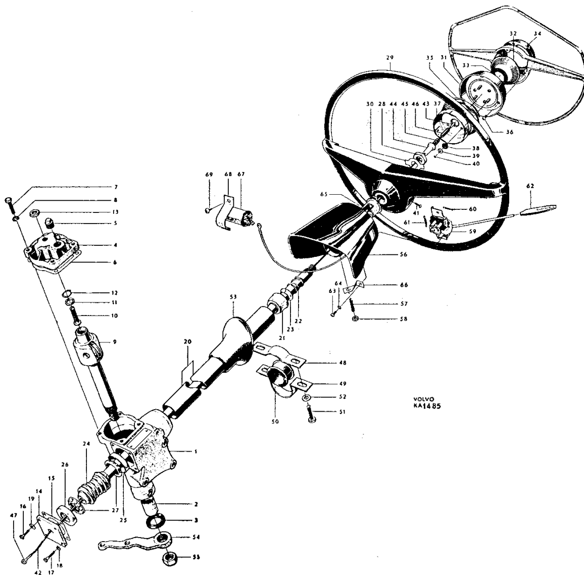
Bild nr 37 Styrinrättning
