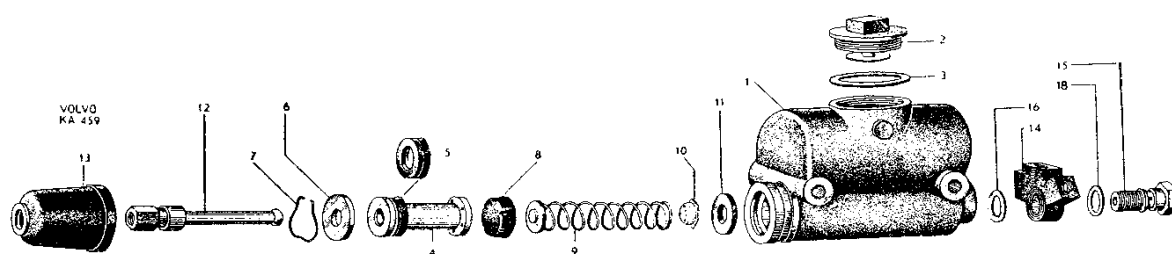
Bild nr 35 Tryckpump
