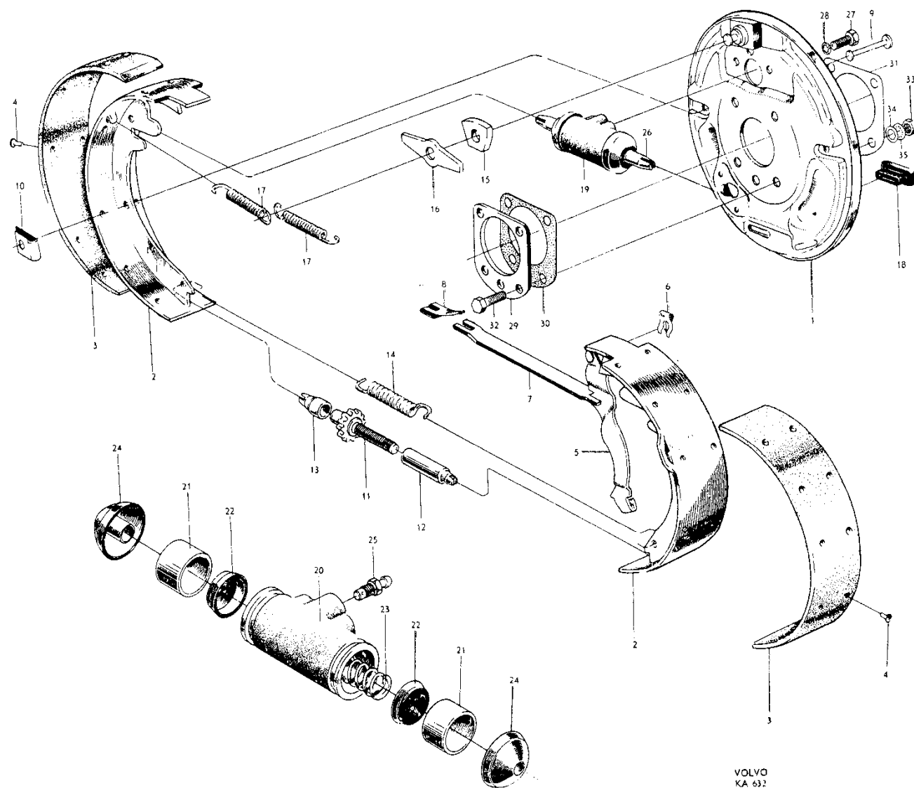
Bild nr 33 Bromsdetaljer för bakhjul
