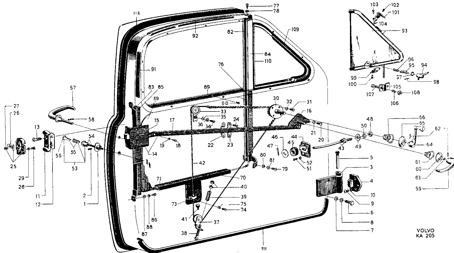
Bild nr 45 Dörrar
