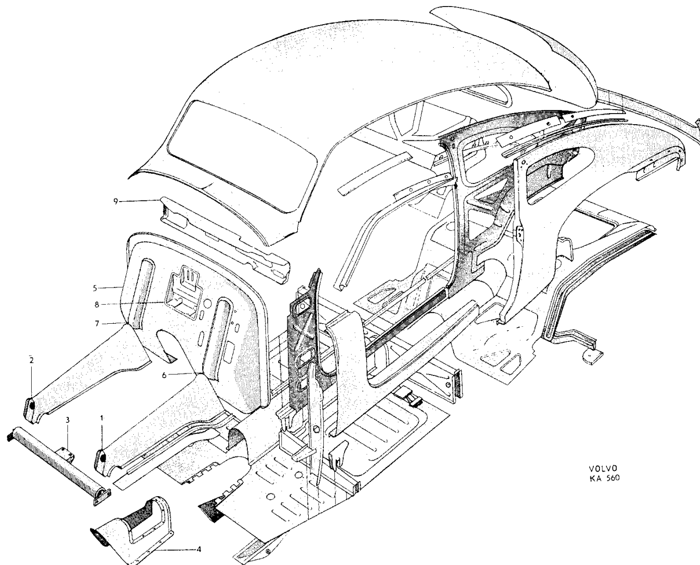
Bild nr 42 Karosseri
