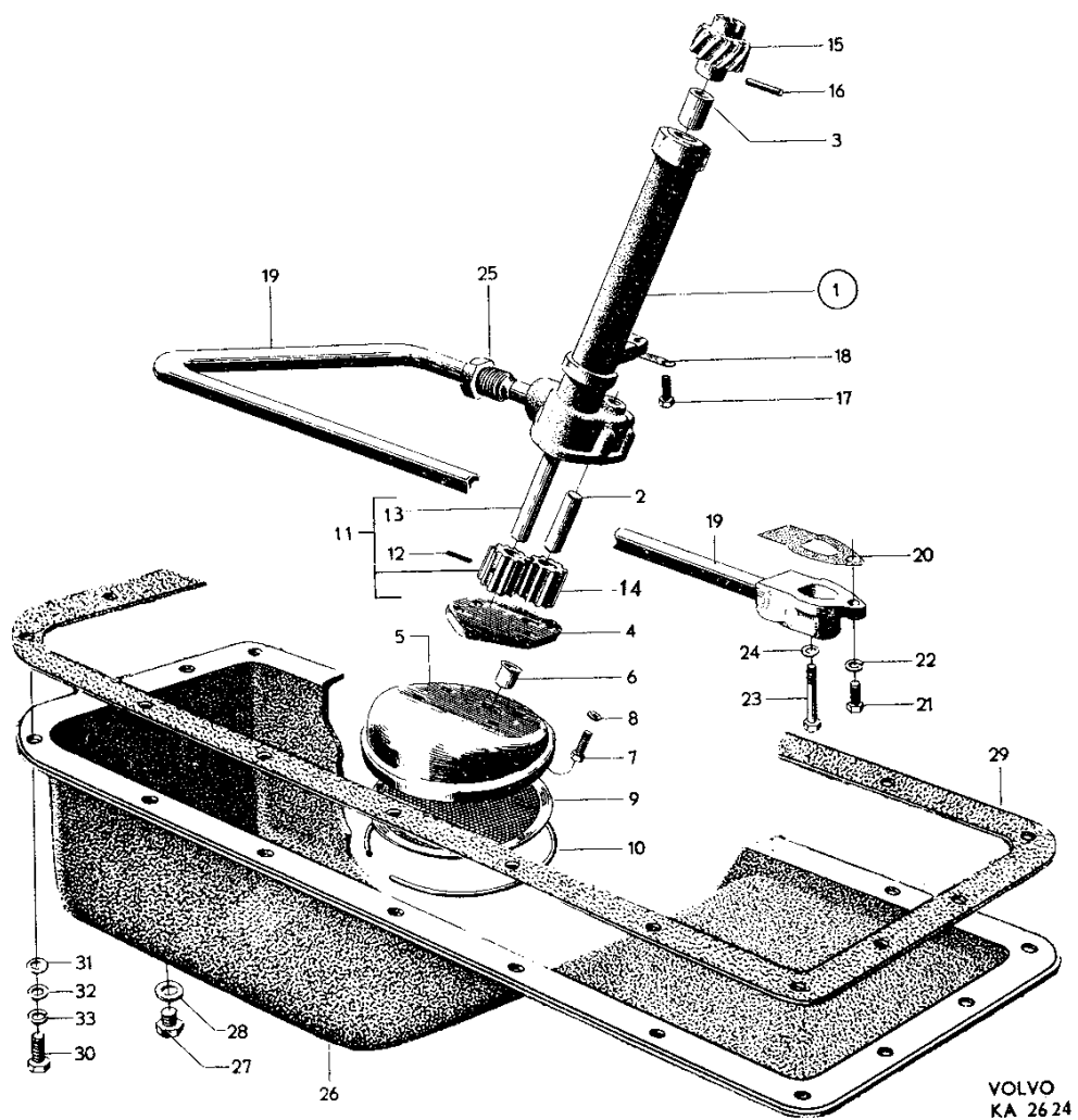
Bild nr 6 Oljepump och oljesump
