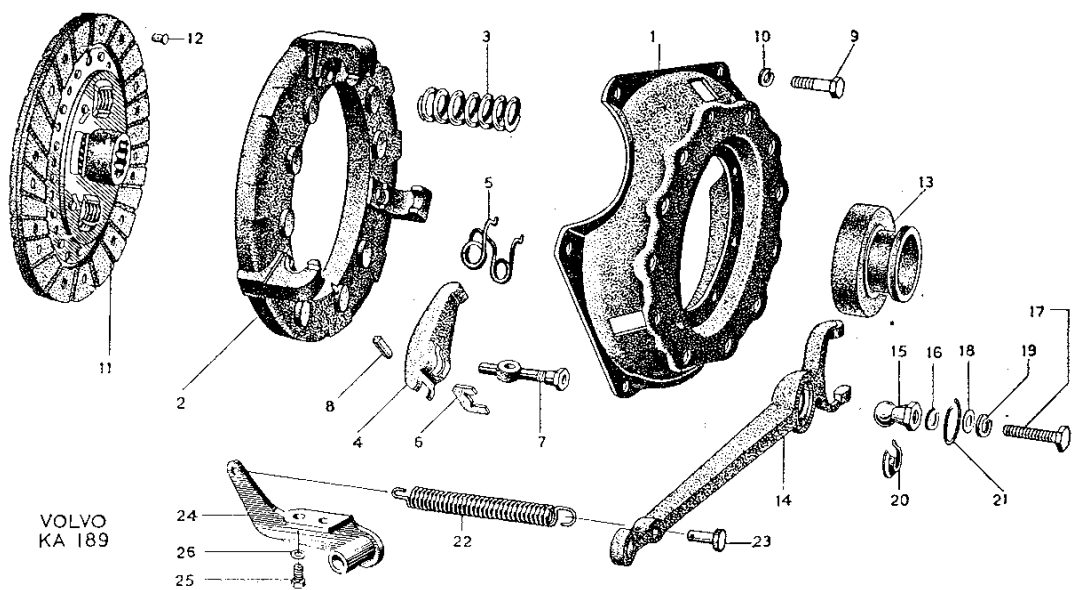
Bild nr 21 Koppling
