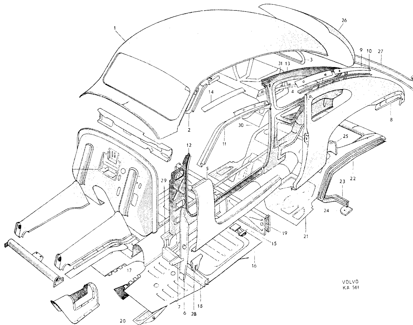
Bild nr 44 Karosseri
