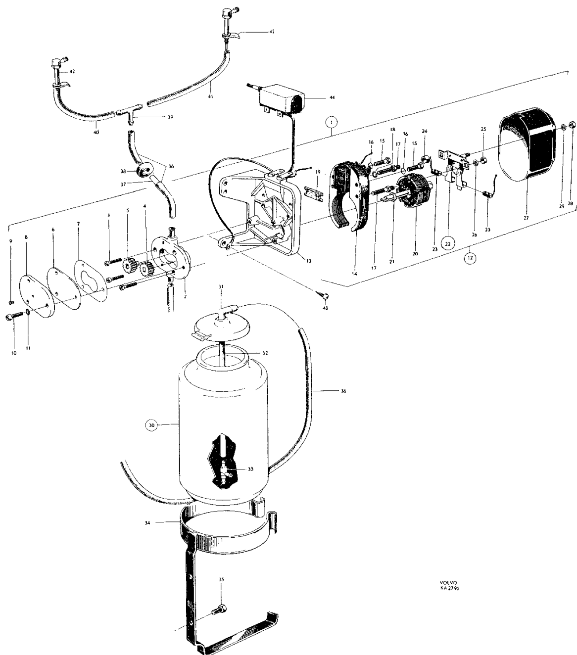
Bild nr 16 Vindrutespolare
