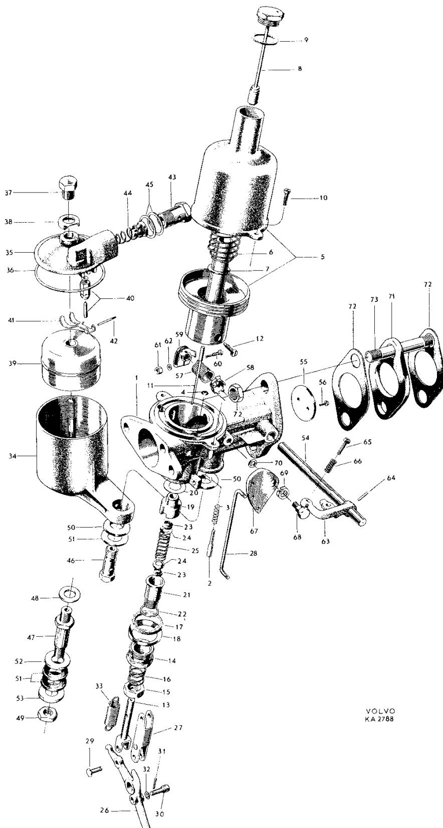
Bild nr 19 Förgasare - B 16 B
