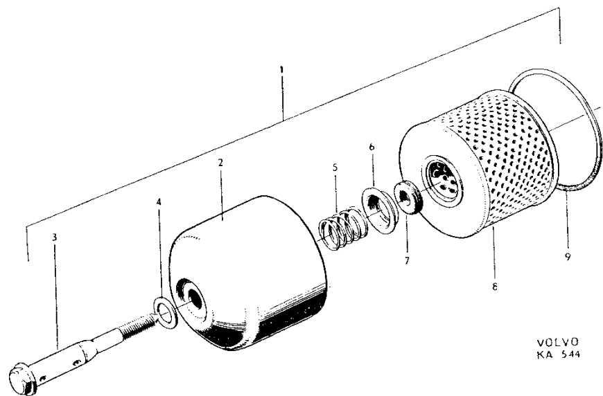
Bild nr 7 Oljefilter, det.nr 403910
