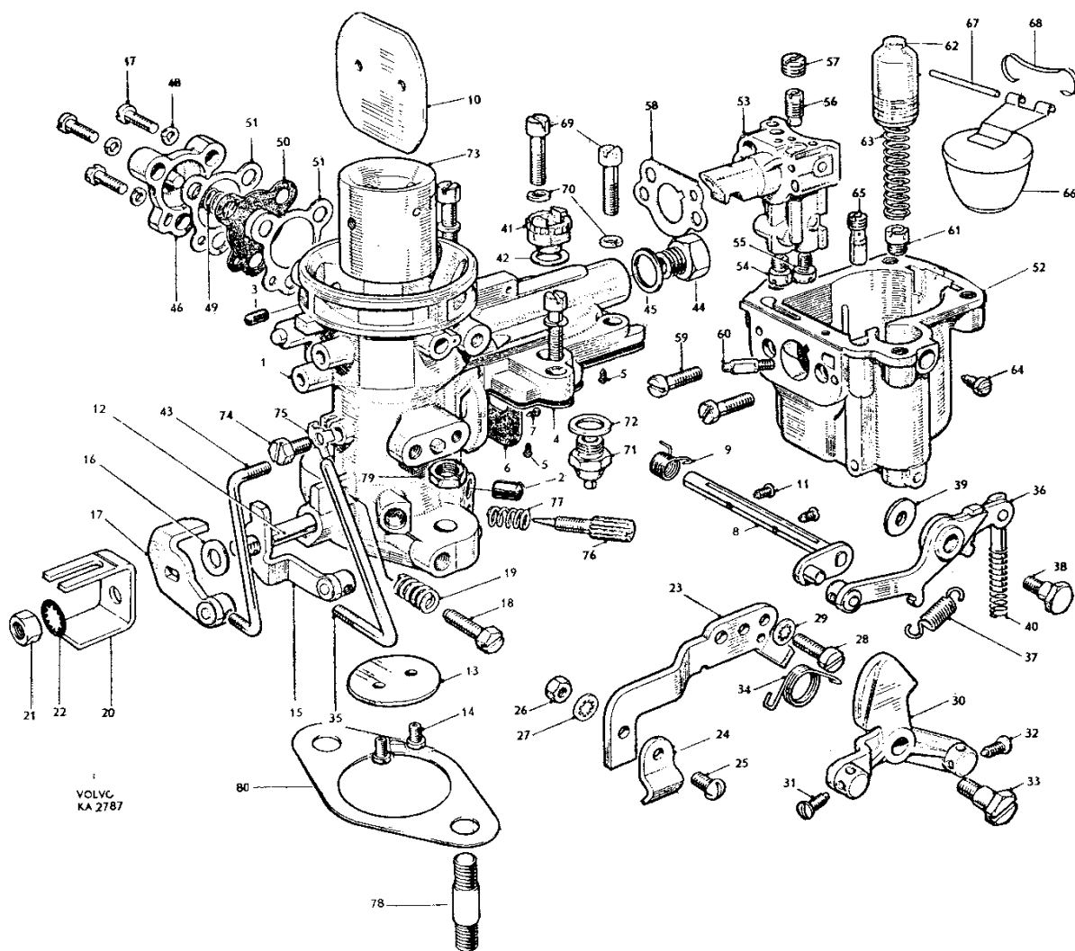
Bild nr 18 Förgasare - B 16 A
