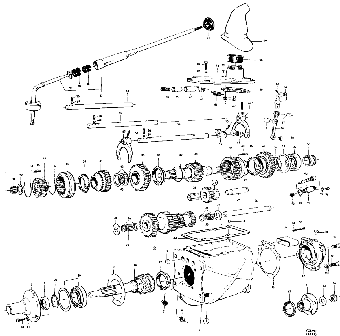
Bild 24b. Væxellåda M40
