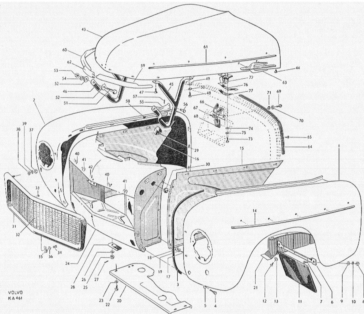
Bild nr 40 Plåtdetaljer på karosseri
