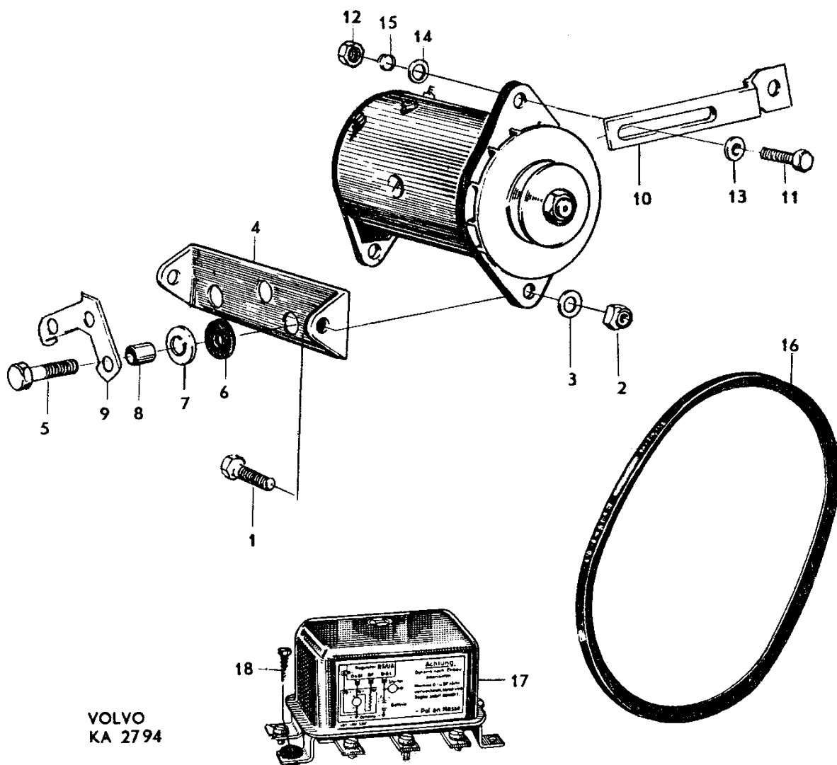
Bild nr 11 Generator
