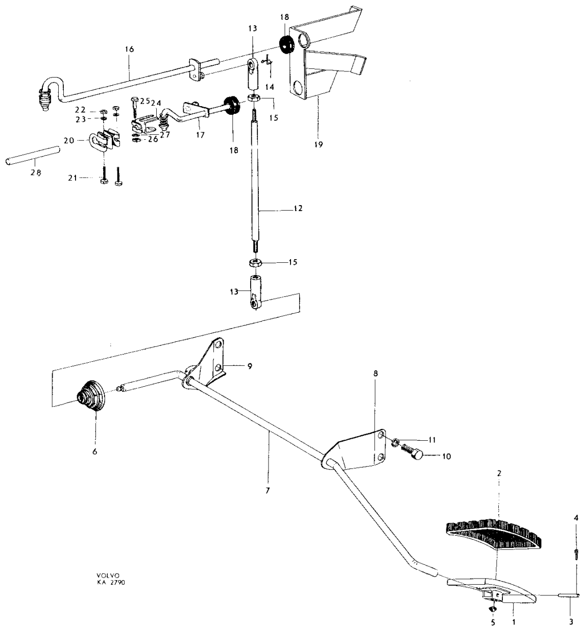
Bild nr 38 Gasreglage
