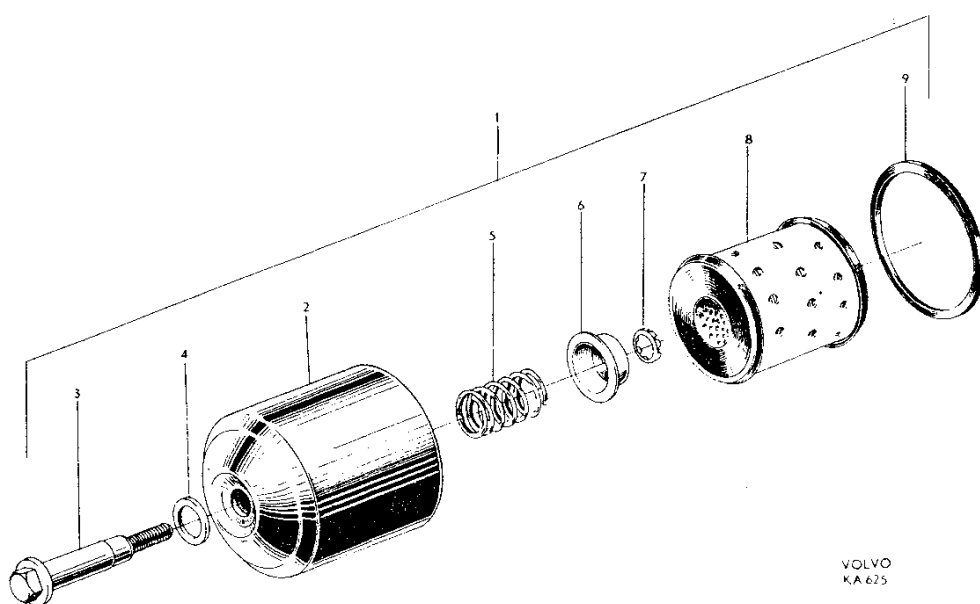
Bild nr 8 Oljefilter, det.nr 418026
