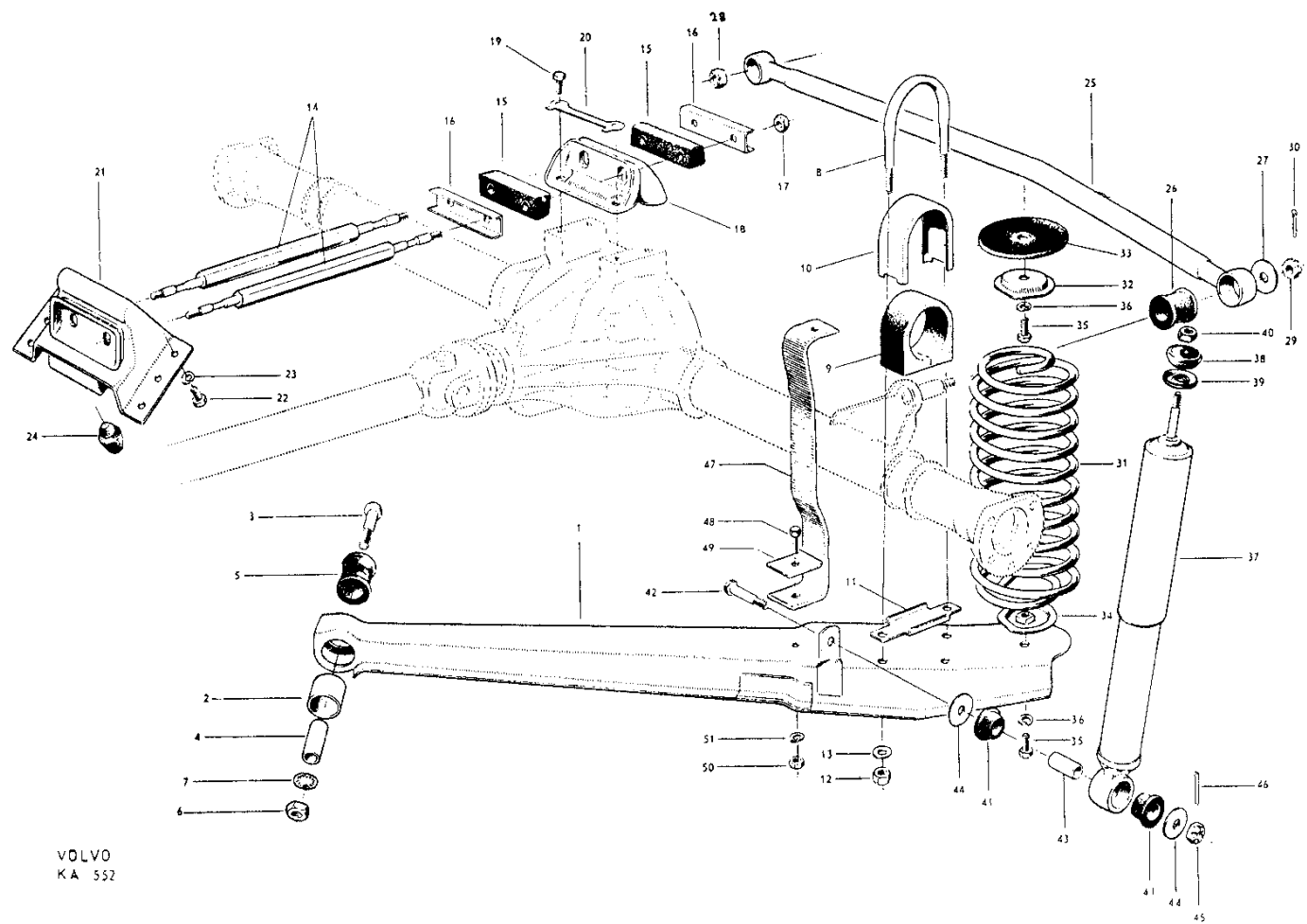
Bild nr 29 Bakaxelupphängning
