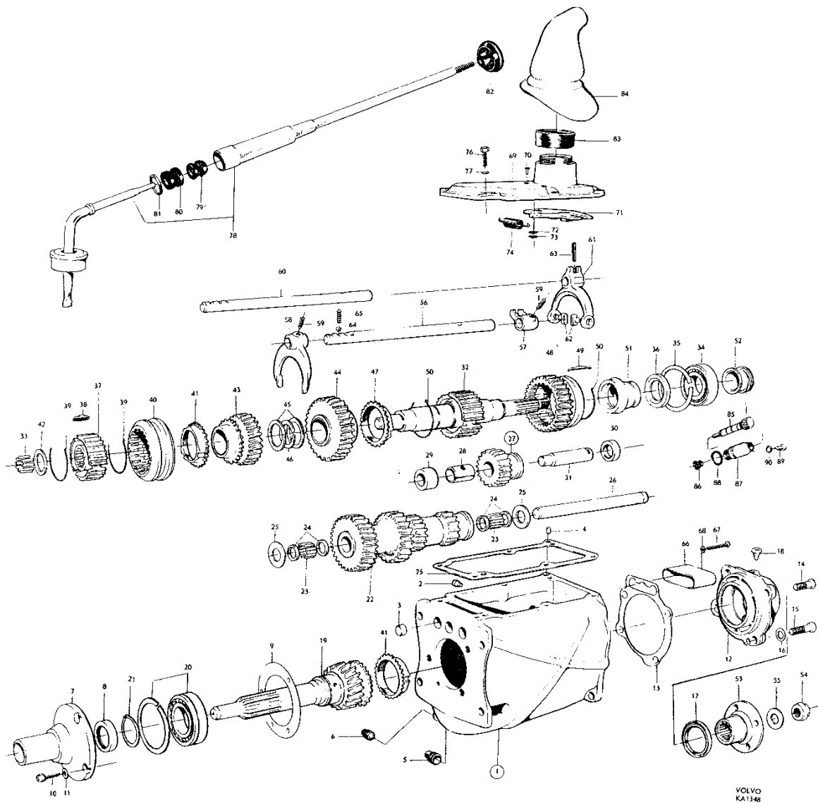
Bild 24a. Vöxellåda M30
