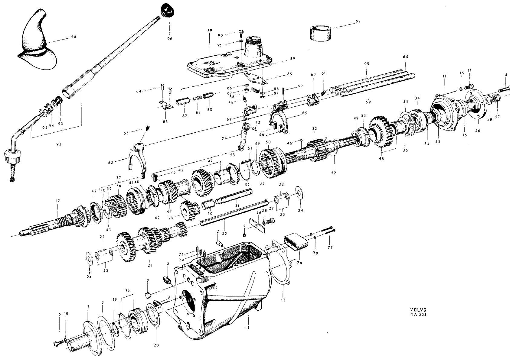
Bild nr 24 Växellåda M 4
