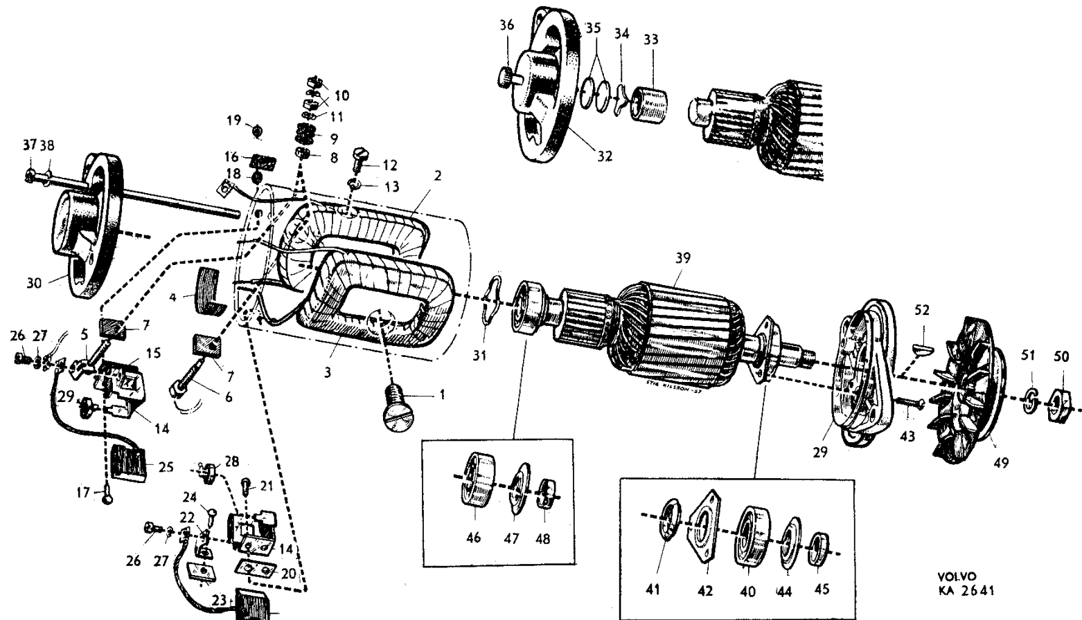
Bild nr 11a Generator
