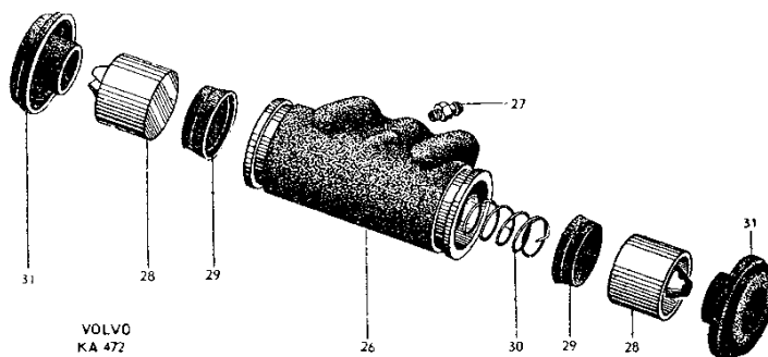
Bild nr 32 Bromsdetaljer för bakhjul
