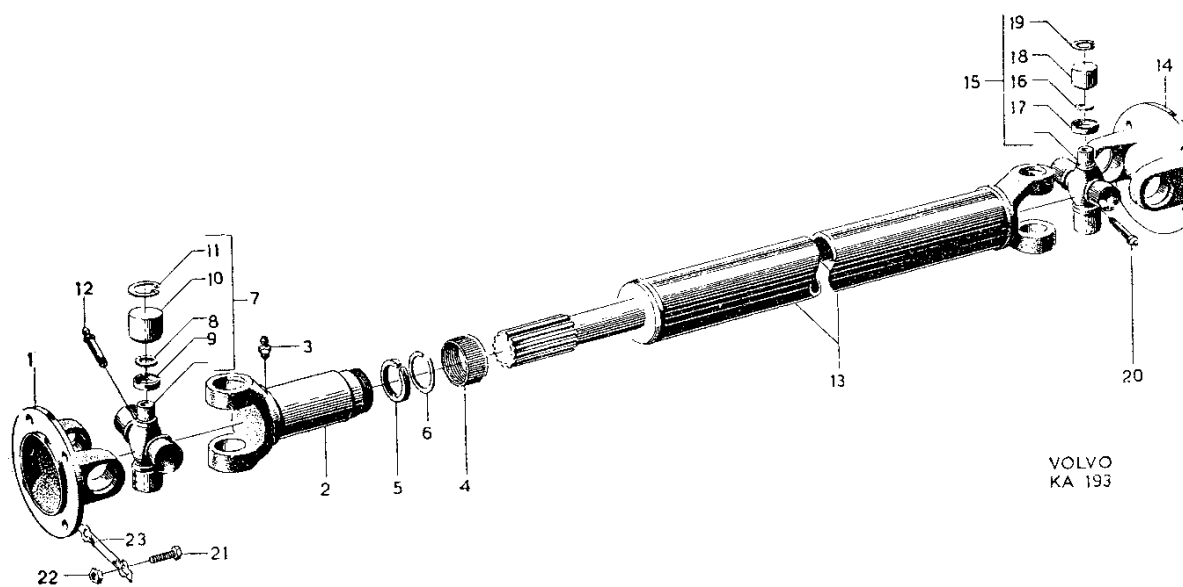
Bild nr 25 Kardanaxel, främre
