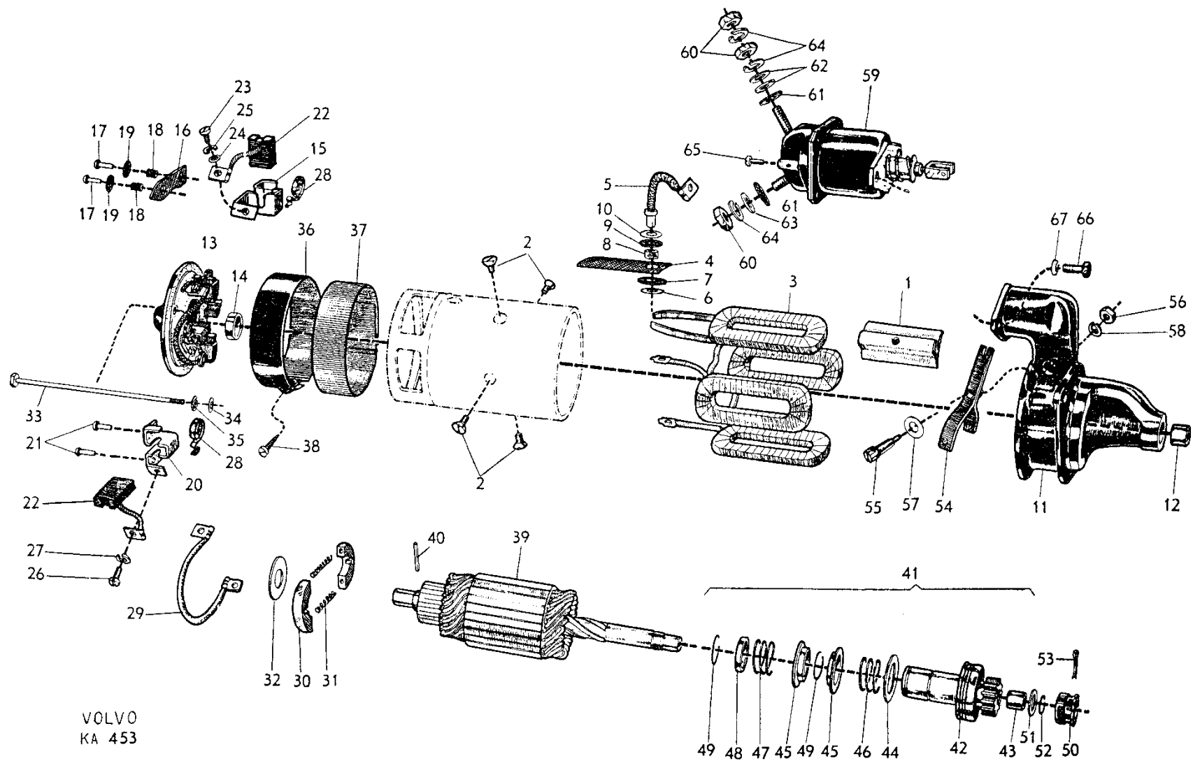
Bild nr 12. Startmotor
