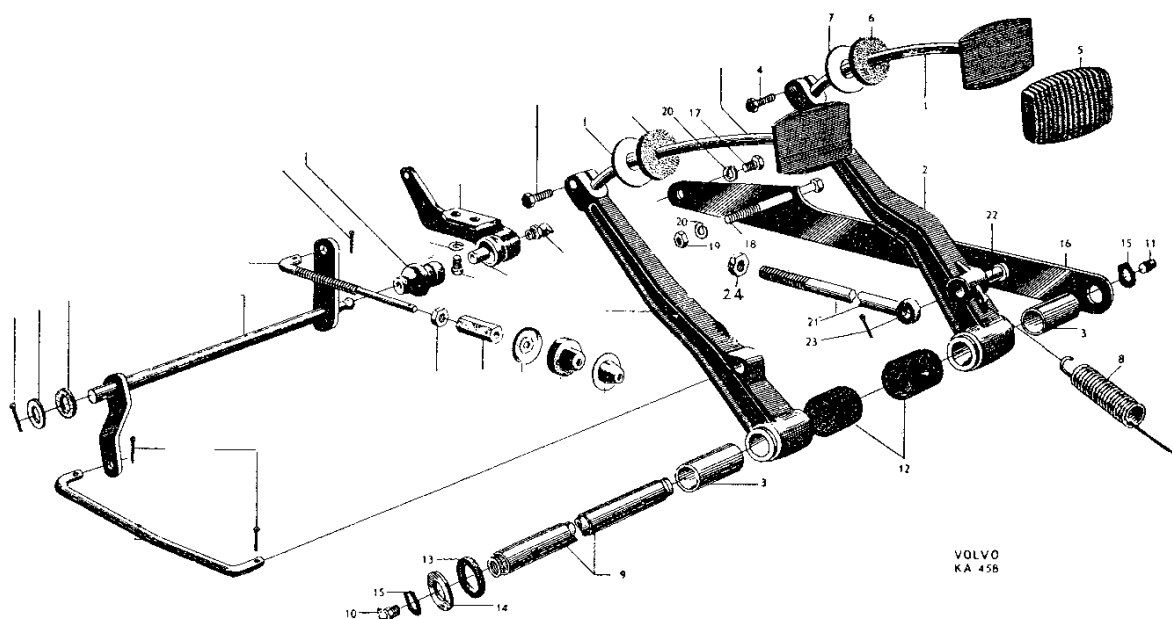
Bild nr 34 Fotbromsmanövrering
