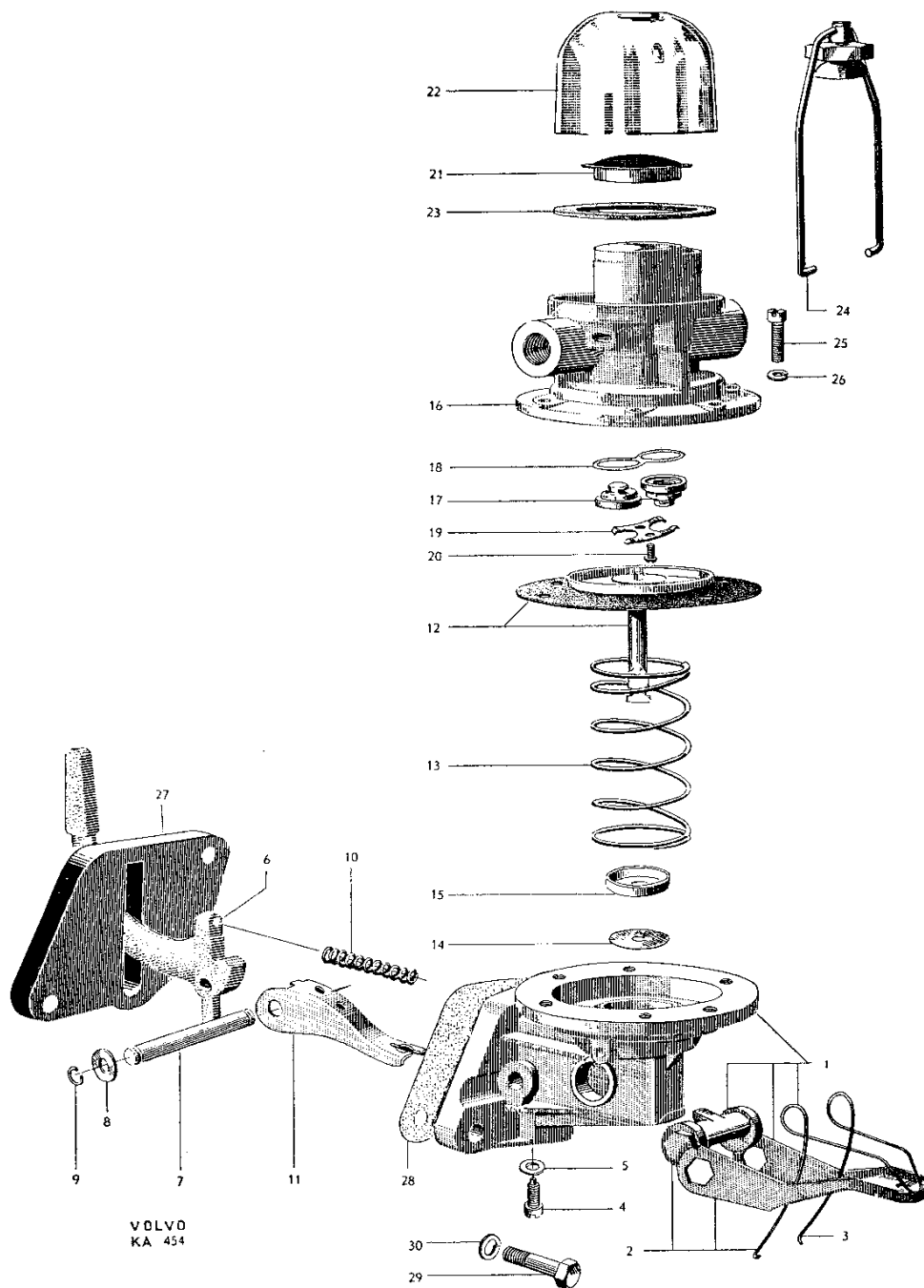
Bild nr 17. Bensinpump
